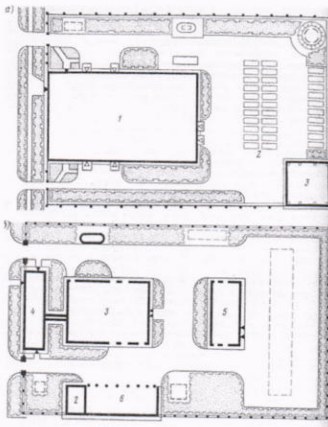
Рис. 7.1. Генеральный план базы на 50 и 100 машин:
