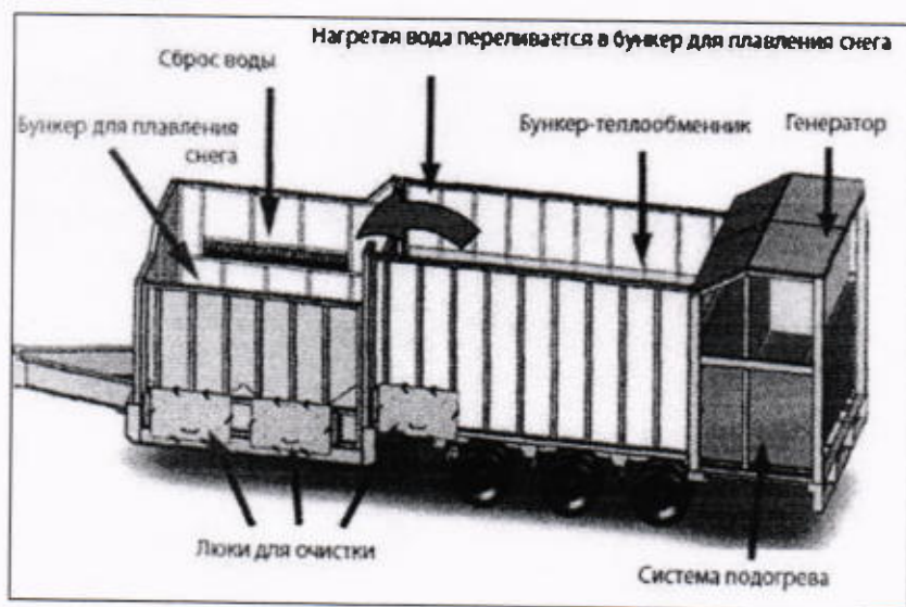
Рис. 6.4. Схема работы снегоплавильной установки
